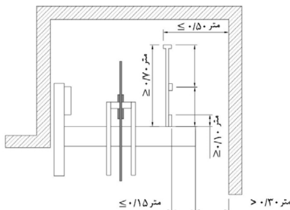
۱- نصب نرده با حداقل ارتفاع ۷۰ سانتی متر و محافظ پا با حداقل ارتفاع ۱۰ سانتی متر الزامی است
