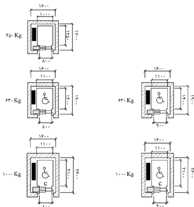
شکل ۵-۱۶- ایجاد چاهک برای آسانسور کششی - اصطکاکی با موتورخانه
