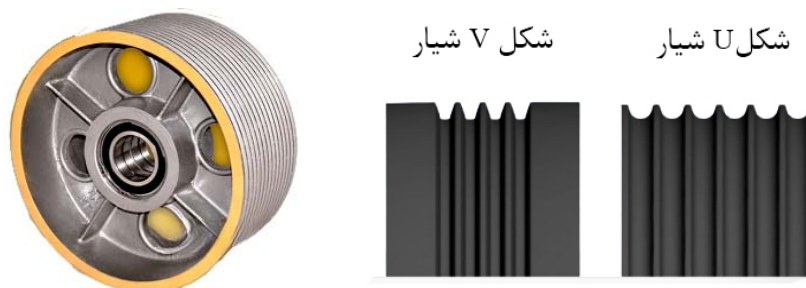
شکل ۶-۳- فلکه کششی و هرزگرد اسانسور کششی.
