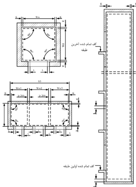
شکل ۵-۱۴- خطوط شاقولی و محدوده رواداری (K)
