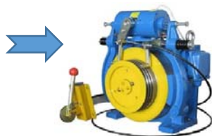
شکل ۶-۳۱- نمونه‌ای از ترمز الکترومگنت الکتروموتور محرک
