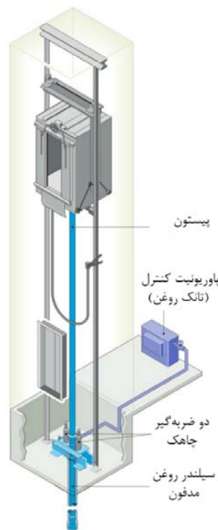
شکل ۳-۵ - آسانسور هیدرولیک جک در زیر-مستقیم
