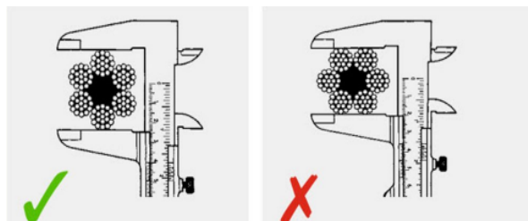
شکل ۸-۳- نحوه صحیح اندازه گیری قطر سیم بکسل ها به وسیله کولیس
